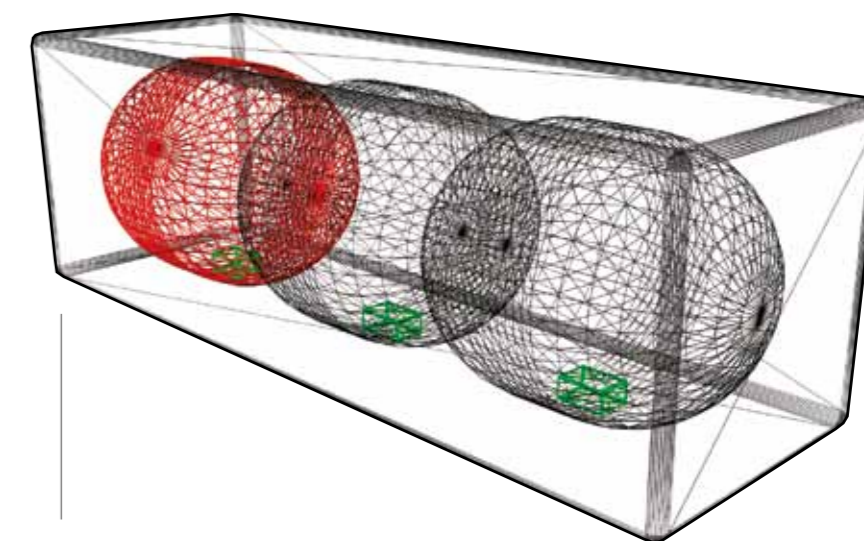
Campo magnetico della vasca. Bathtub's magnetic field. Champ magnétique de la baignoire. Campo magnético de la bañera.
