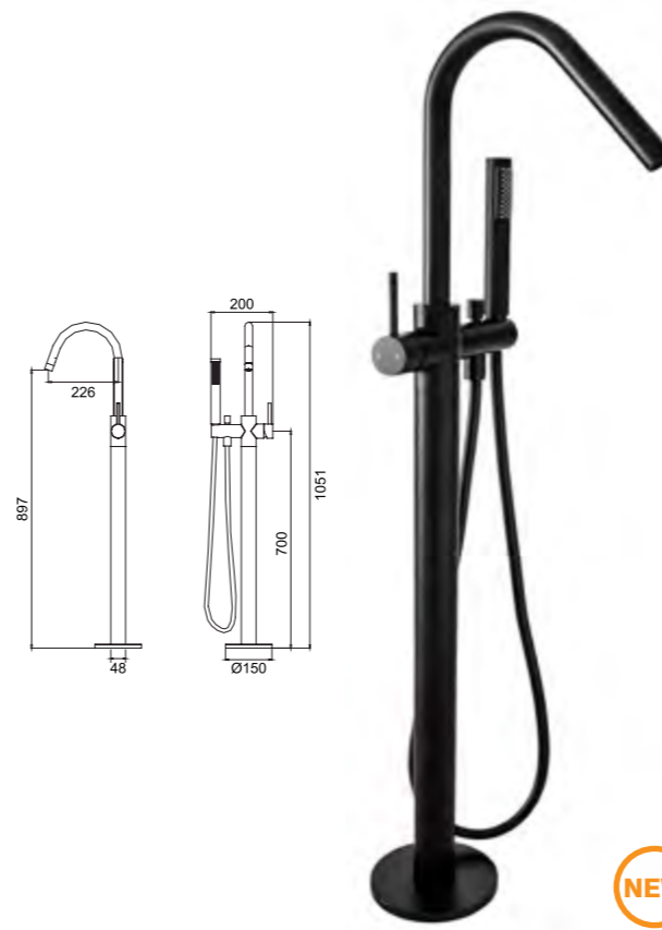
RTSE4007828 TA55/650 8,1 Kg 0,084 m³
