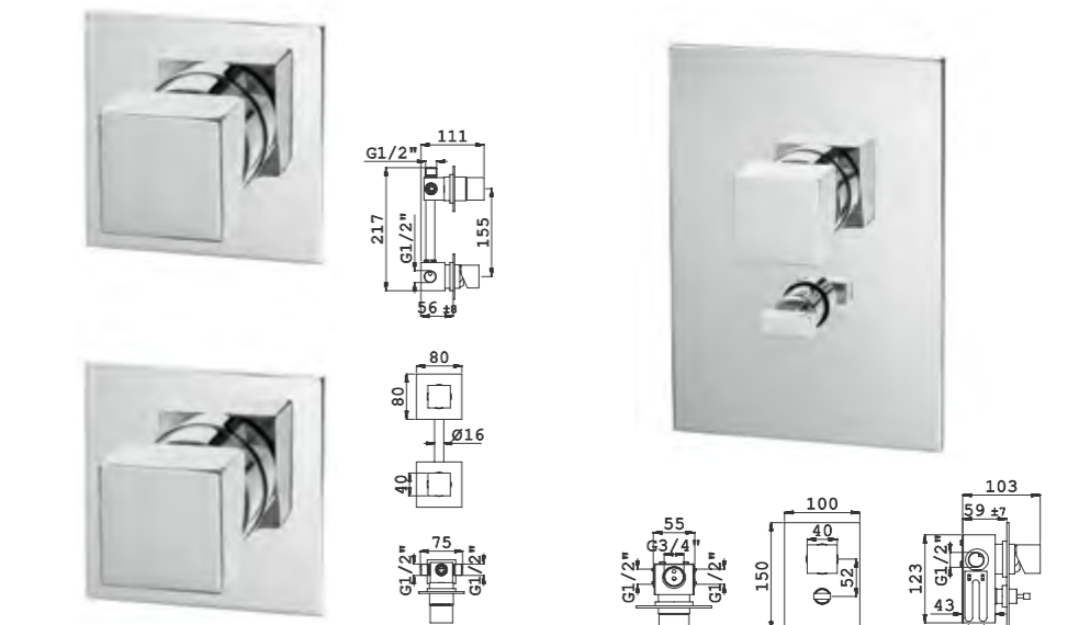
RTQUAD090A TA36/230 2,5 Kg 0,01 m 3 3 vias - 3 ways 3 voies - 3 wege 3 vias
