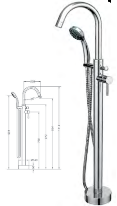
RT080930 TA51/500 8,1 Kg 0,09 m³
