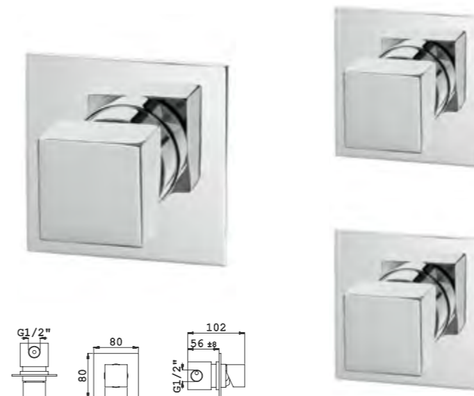
RTQUAD090 TA18/110 1,8 Kg 0,01 m 3 1 via - 1 way 1 voie - 1 wege 1 via
