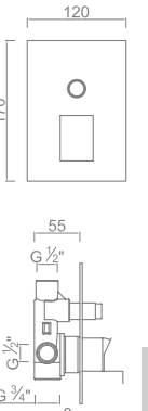
RTUX006 2 vias - 2 ways 2 voies - 2 wege 2 vias TA28/175 2,3 Kg 0,01 m³
