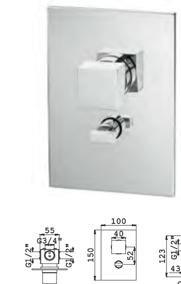
RTQUAD090A TA36/230 2,5 Kg 0,01 m 3 3 vias - 3 ways 3 voies - 3 wege 3 vias
