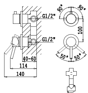
RT10716011 TA26/165 2,60 Kg 2 vias - 2 ways 2 voies - 2 wege - 2 vias 0,006 m³
