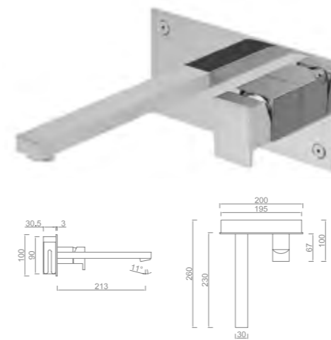
RTUX008 TA32/200 9 Kg 0,03 m³
