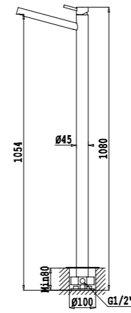
RT10779011E TA57/730 14 Kg 0,02 m 3
