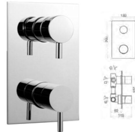
RTGRS07/1 3 vias - 3 ways - 3 voies 3 wege - 3 vias TA38/250 2 Kg 0,006 m 3
