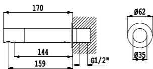
RT13000171 TA43/300 2,20 Kg 0,005 m 3
