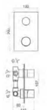
RTGRS07/1 3 vias - 3 ways - 3 voies 3 wege - 3 vias TA38/250 2 Kg 0,006 m 3
