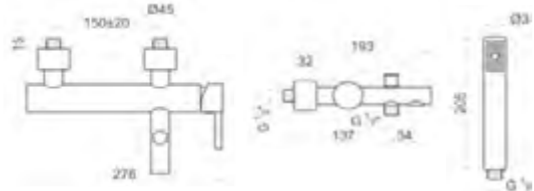
RTGRS03 TA33/210 2,9 Kg 0,008 m 3
