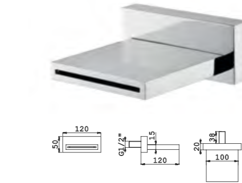
RTCASC060 TA31/190 2 Kg 0,001 m 3
