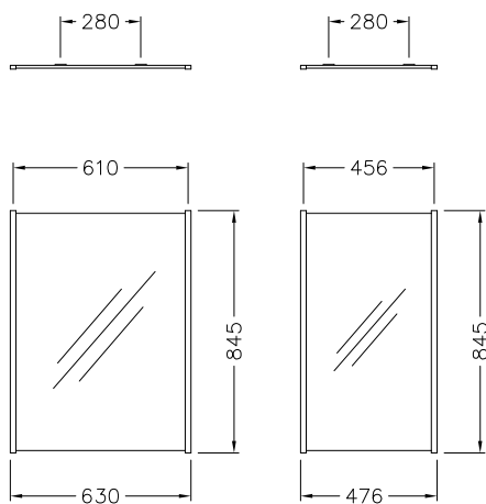
AU: 115058 NZ: 586162 610mm AU: 115057 NZ: 586163 456mm Loure mirror: pg. 96
