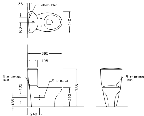
AU: 059994 NZ: 507153 Presqu'île™ close coupled toilet: pg. 29
