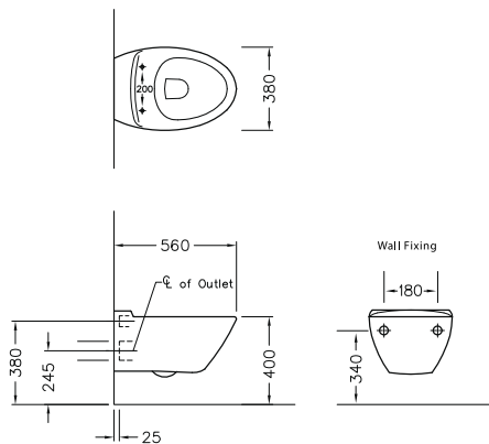
AU: 115456 NZ: 585990 Presqu'île™ wall-hung toilet: pg. 31
