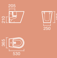
BIDET BTW
