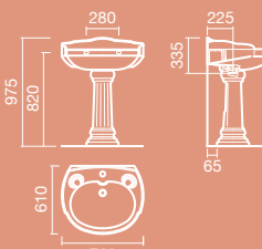
WASHBASIN 70
