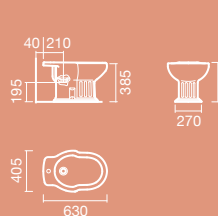
BIDET simple
