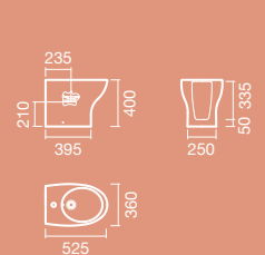
BIDET BTW
