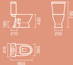
TOILET compact
