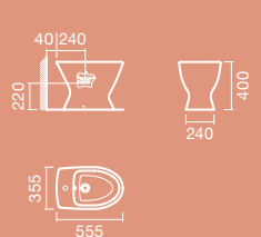
BIDET simple
