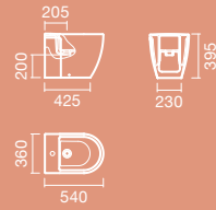
BIDET BTW
