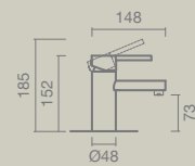
WASHBASIN
