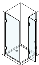
SHOWER ENCLOSURE W/ 1 DOOR + 1 FIXED PANEL + 1 SIDE PANEL (SIDE CLOSING) PAROIS DE DOUCHE A/ 1 PORTE + 1 PAN. FIXE + 1 PANNEAU LATÉRAL (FERMETURE LATÉRAL) MAMPARA DE DUCHA C/ 1 PUERTA + 1 PANEL FIJO + 1 PANEL LATERAL (CIERRE LATERAL)
