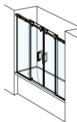
BATH ENCLOSURE W/ 2 SLIDING DOORS + 2 FIXED PANELS PARE-BAIGNOIRE A/ 2 PORTES COLISSANTES + 2 PANNEAUX FIXES MAMPARA DE BAÑO C/ 2 PUERTAS CORREDERAS + 2 PANELES FIJOS
