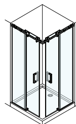
SHOWER ENCLOSURE W/ 2 SLIDING DOORS + 2 FIXED PANELS PAROIS DE DOUCHE A/ 2 PORTES COULISSANTES + 2 PANNEAUX FIXES MAMPARA DE DUCHA C/ 2 PUERTAS CORREDERAS + 1 PANELES FIJOS
