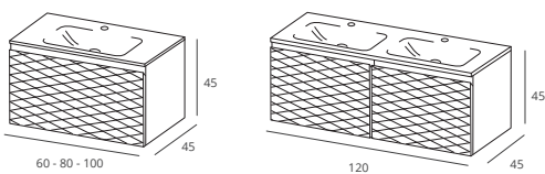
BASE UNIT WITH DRAWERS + INTERIOR DRAWERS MEUBLE AVEC TIROIRS + TIROIRS INTÉRIEURS MUEBLE CON CAJONES + CAJONES INTERIORES
