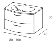
SUSPENDED BASE UNIT WITH 2 DRAWERS AND COUNTERTOP WASHBASIN MEUBLE SUSPENDU AVEC 2 TIROIRS ET LAVABO MUEBLE SUSPENDIDO CON 2 CAJONES Y LAVABO
