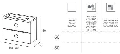
BASE UNIT W/ 2 DRAWERS AND ZIP COUNTERTOP WASHBASIN MEUBLE AVEC 2 TIROIRS ET LAVABO ZIP MUEBLE CON 2 CAJONES Y LAVABO ZIP
