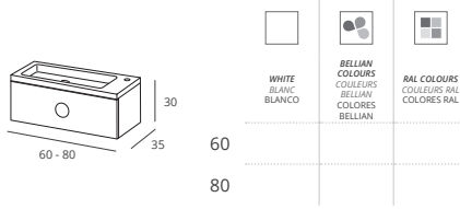
SUSPENDED BASE UNIT W/ 1 DRAWER AND ZIP COUNTERTOP W. MEUBLE SUSPENDU AVEC 1 TIROIR ET LAVABO ZIP MUEBLE SUSPENDIDO CON 1 CAJÓN Y LAVABO ZIP
