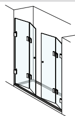
SHOWER ENCLOSURE W/ 2 FOLDING DOOR S PAROIS DE DOUCHE A/ 2 PORTES PLIANTES MAMPARA DE DUCHA C/ 2 PUERTAS PLEGABLES
