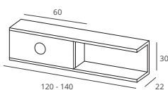
SHELF WITH 1 DOOR ÉTAGÈRE AVEC 1 PORTE ESTANTE CON 1 PUERTA
