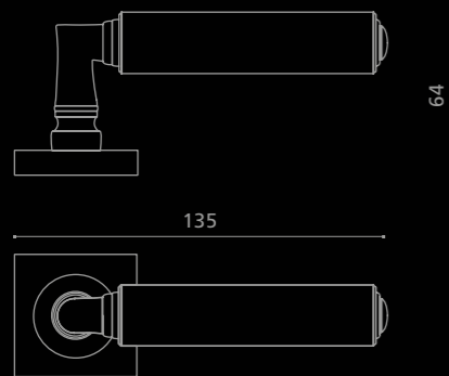
CUBET36F1OP9WC Maniglia in cristallo bianco latte, molato a mano con mole a pietra. Montatura in ottone lucido con nottolino WC. Hand bevelled in stone, white crystal door handle. Polished brass base with WC key set.
