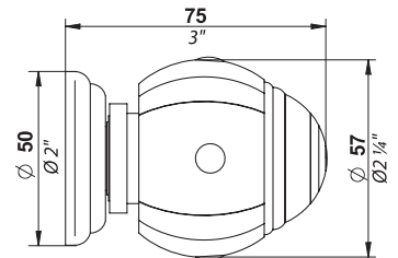
2 Poignée de porte Door handle Türknohf
