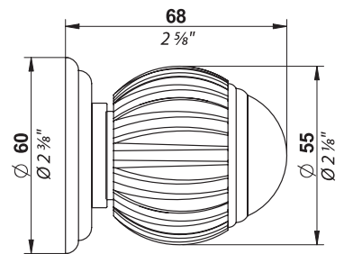
❶ Bouton grand modèle Door knob Grosser Knopf
