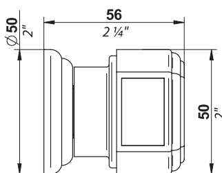
❷ Poignée de porte Door handle Türknoopf
