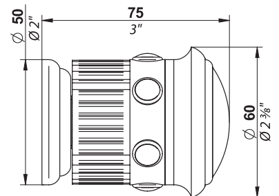
❷ Poignée de porte Door handle Türknohf
