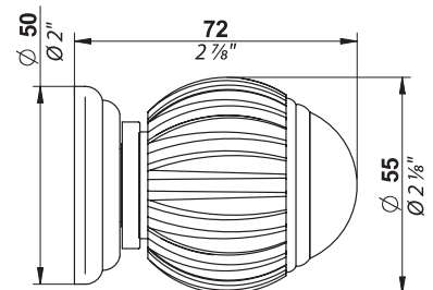
❷ Poignée de porte Door handle Türknohf
