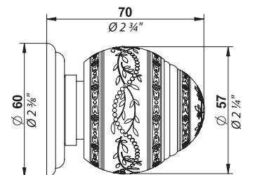
1 Bouton grand modèle Door knob Grosser Knopf
