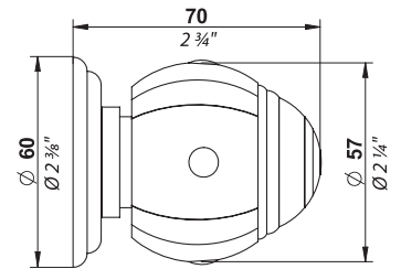
1 Bouton grand modèle Door knob Grosser Knopf
