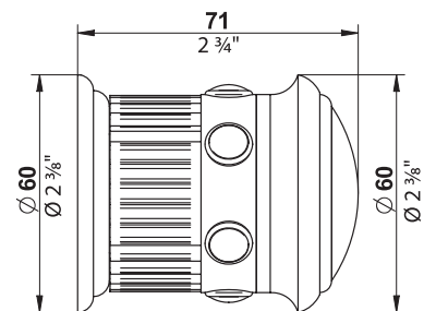
❶ Bouton grand modèle Door knob Grosser Knopf
