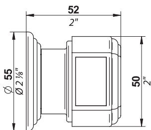
❶ Bouton grand modèle Door knob Grosser Knopf
